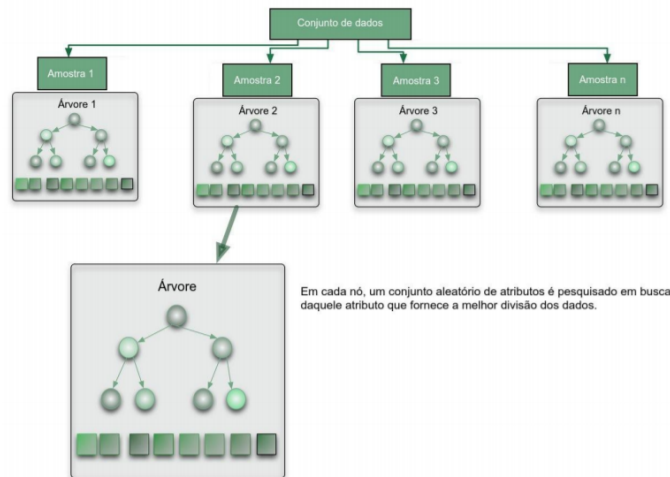
Figura 2 - Representação esquemática do funcionamento do Random Forest
