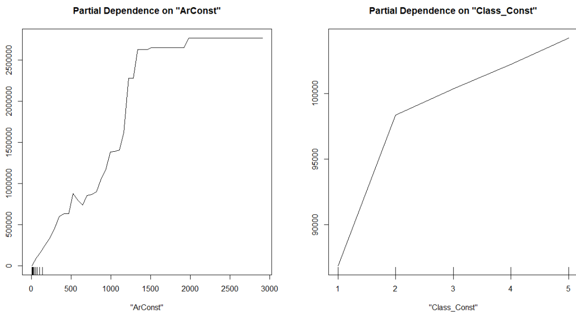
Gráfico 1 - Dependência parcial do preço unitário das construções com o modelo RF.
